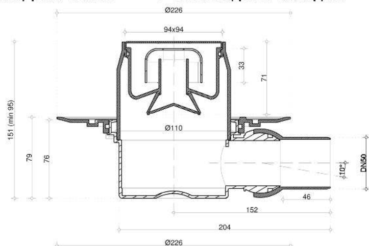
МОДЕЛЬ БАЗЫ: 1 - БАЗА С ОДНИМ ВЫХОДОМ
