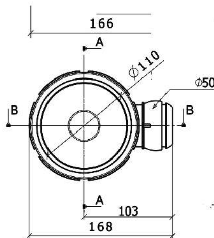
МОДЕЛЬ БАЗЫ: 2 - БАЗА С ОДНИМ ВХОДОМ И ОДНИМ ВЫХОДОМ
