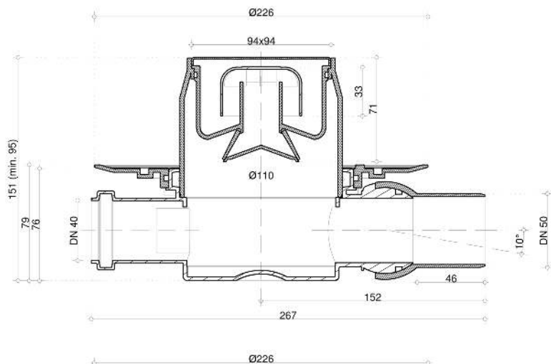
МОДЕЛЬ БАЗЫ: 2 - БАЗА С ОДНИМ ВХОДОМ И ОДНИМ ВЫХОДОМ
