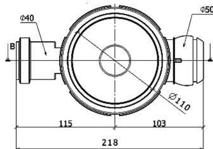
МОДЕЛЬ БАЗЫ: 2 - БАЗА С ОДНИМ ВХОДОМ И ОДНИМ ВЫХОДОМ
